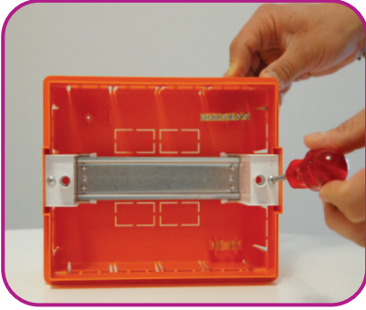
Raylı sistem, vidalar sökülerek kolayca dışarı alınır.
