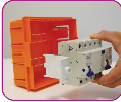
Sigortalar dışarıda rahatça monte edilir.
